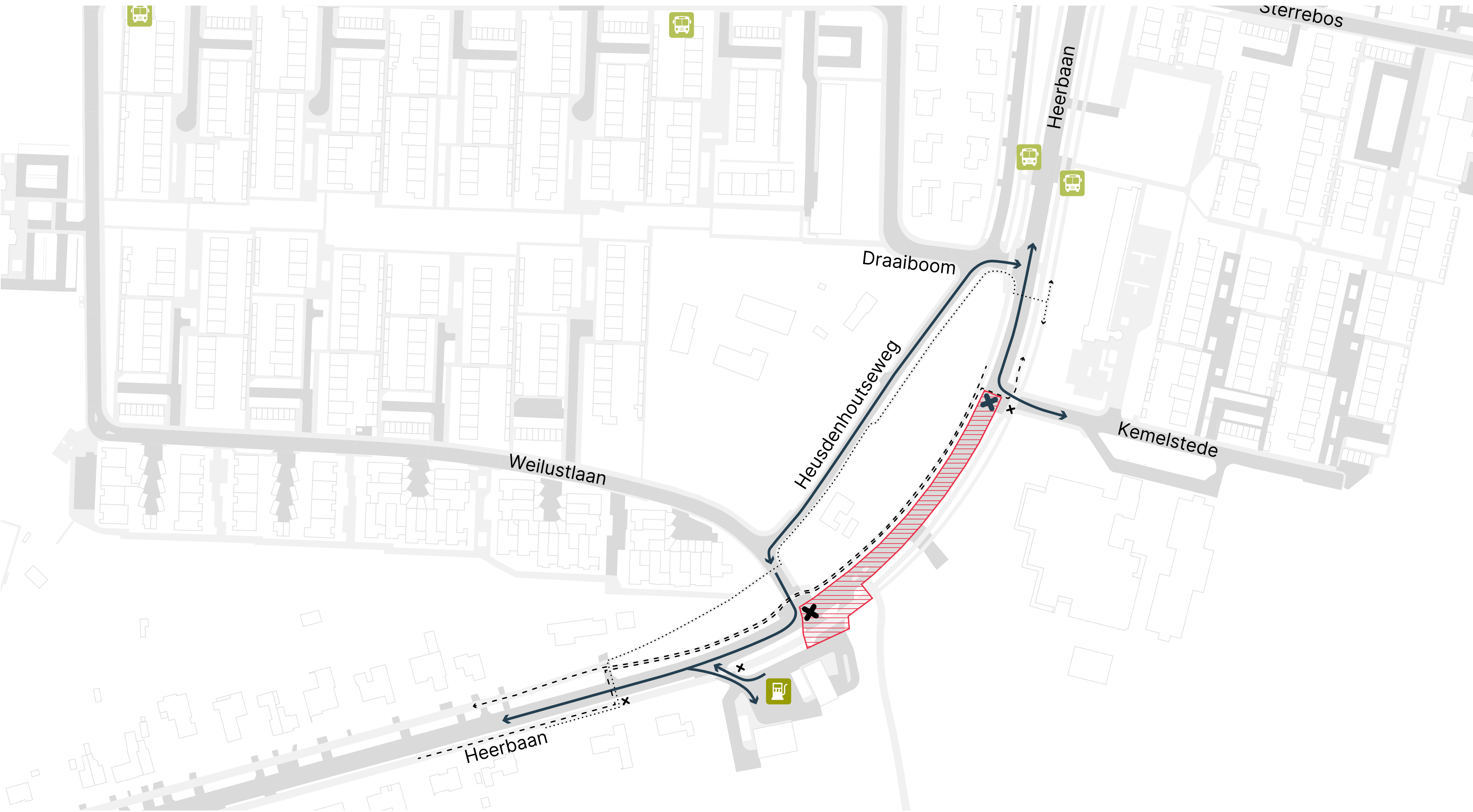
Fase 3.1 - Heerbaan Omleiding mogelijk via Heusdenhoutseweg of volg omleidingsroute P + T. Kemelstede en Weillustlaan bereikbaar.
